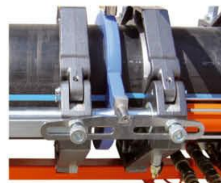
Фиксация нагревателя
