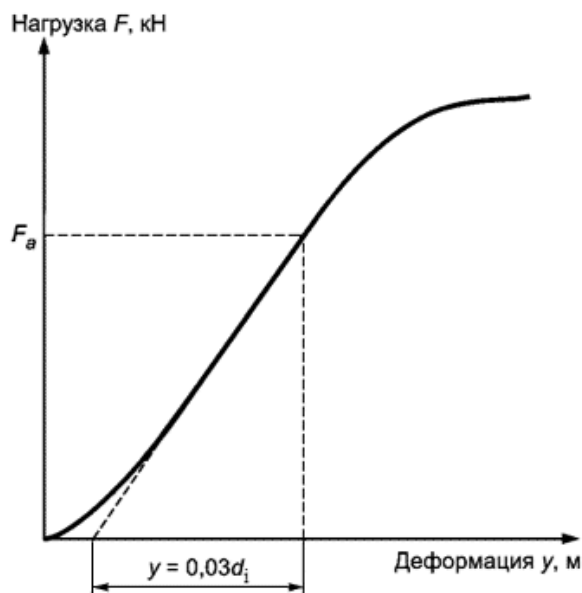
Рисунок В.1 - Кривая "нагрузка-деформация"
